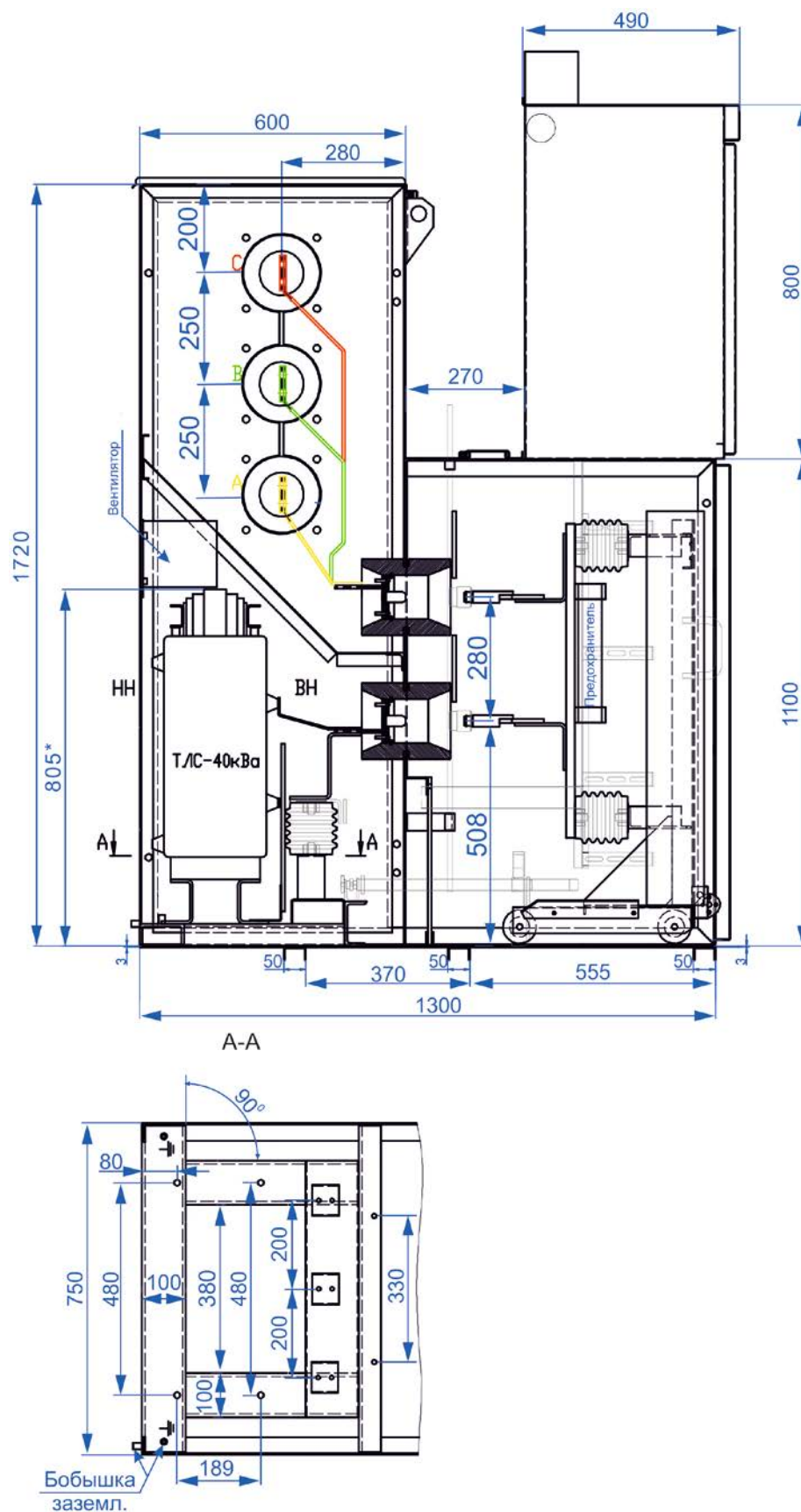
Рисунок 4 - Шкаф ШСТ (с трансформатором собственных нужд)
