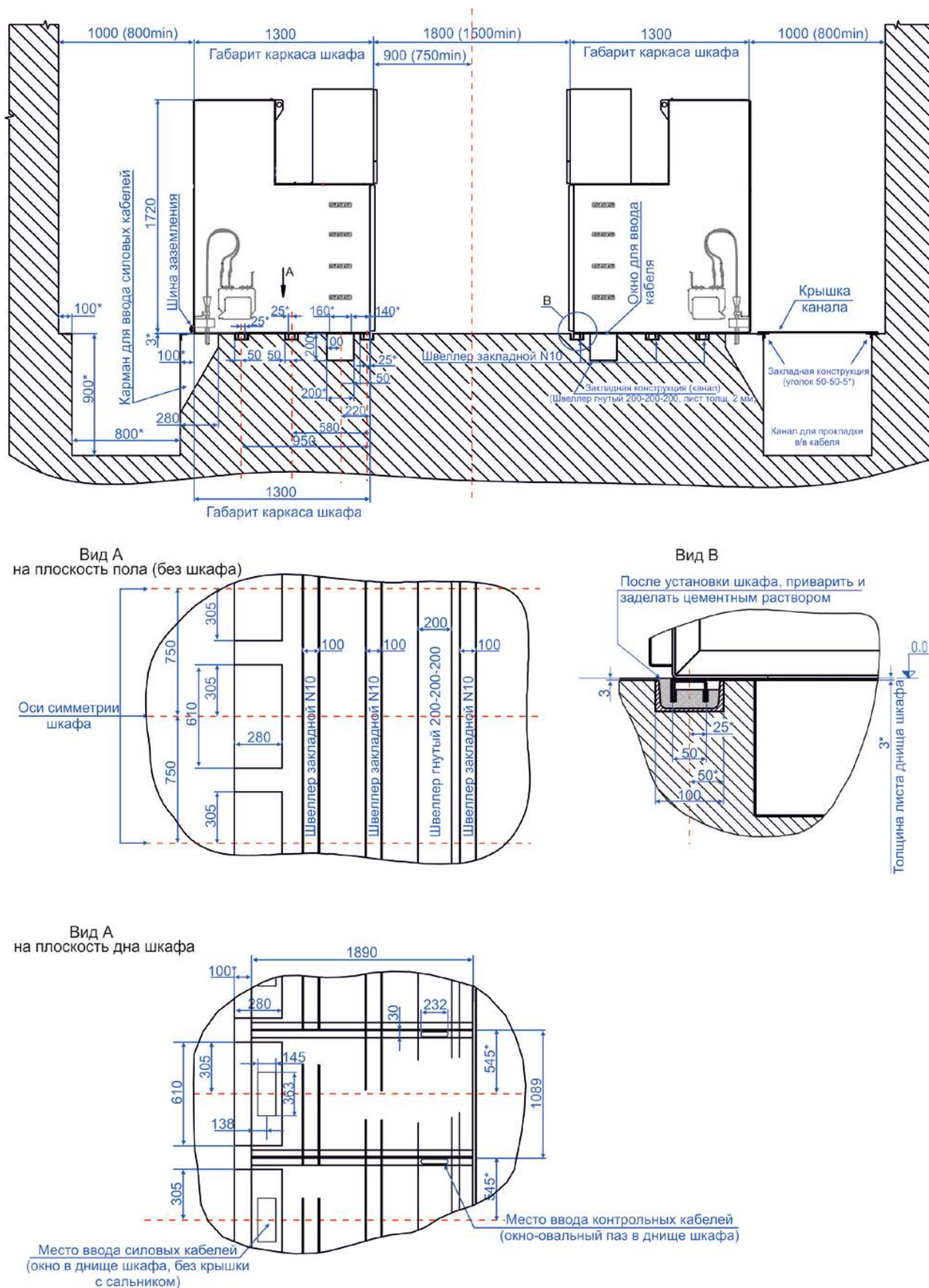
Рисунок 22 - Установка КМ-1КФ в помещении РУ (монтаж и узлы крепления шкафов)
