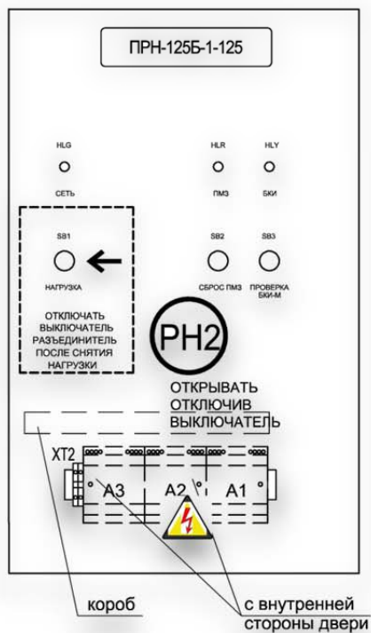
Рисунок 2 Общий вид ПРН с габаритными размерами
