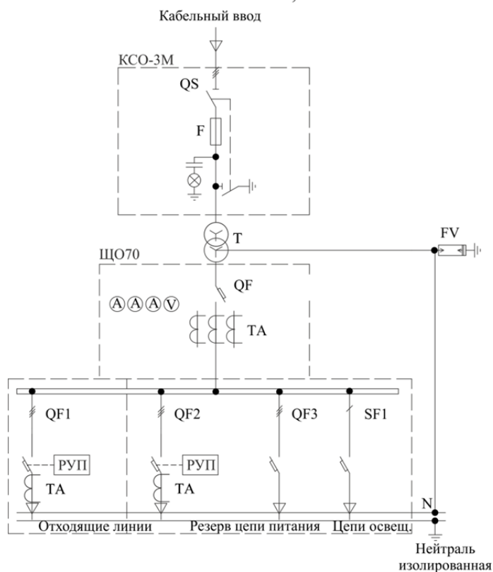
Рисунок 11 КТПН – 630 кВА с кабельным вводом
