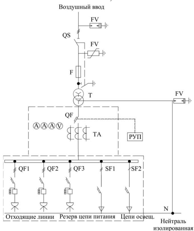
Рисунок 2 КТПН – 63 кВА с воздушным вводом
