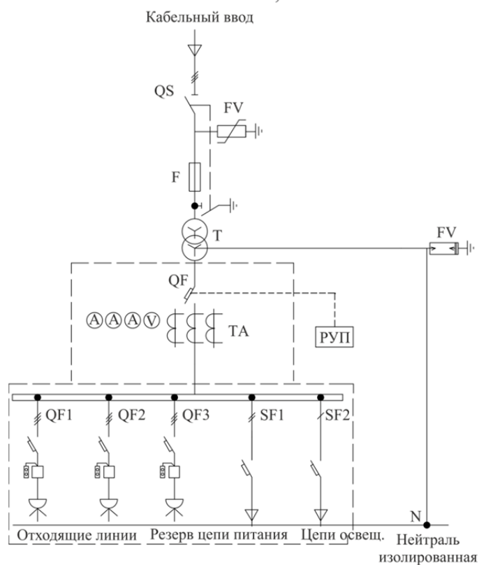
Рисунок 1 КТПН – 63А кВ с кабельным вводом
