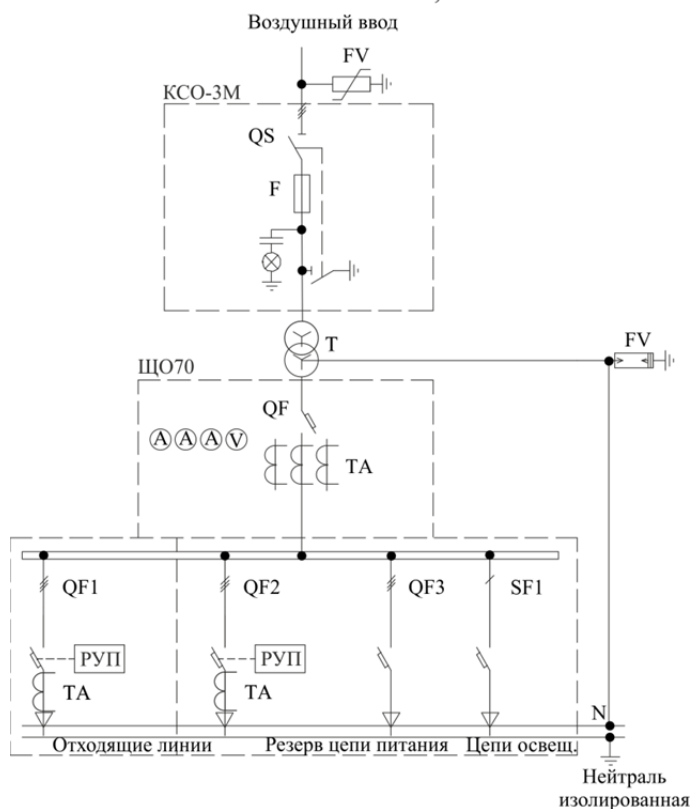
Рисунок 12 КТПН – 630 кВА с воздушным вводом
