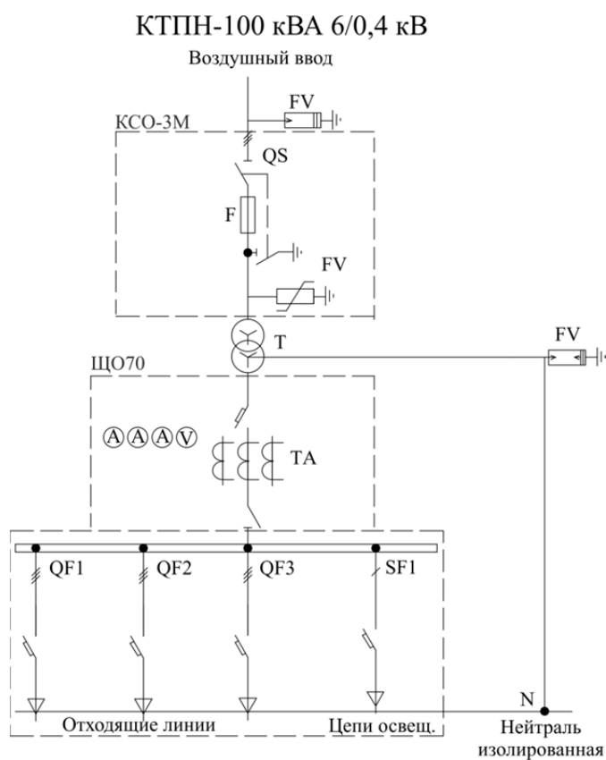
Рисунок 4 КТПН – 100 кВА с воздушным вводом
