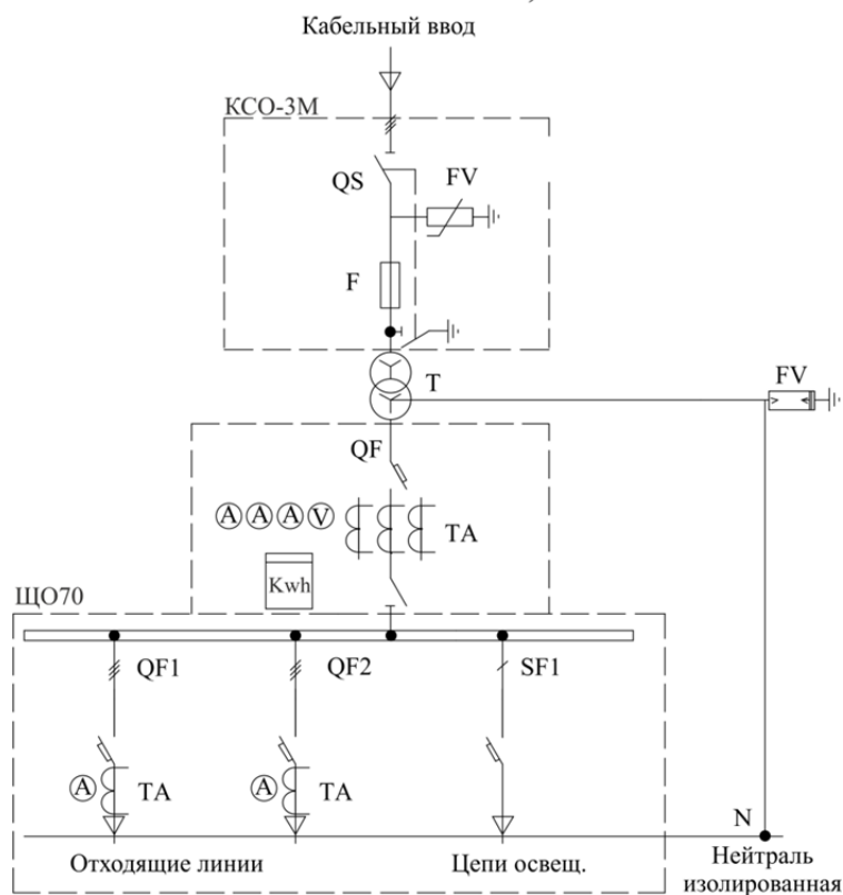
Рисунок 5 КТПН – 160 кВА с кабельным вводом
