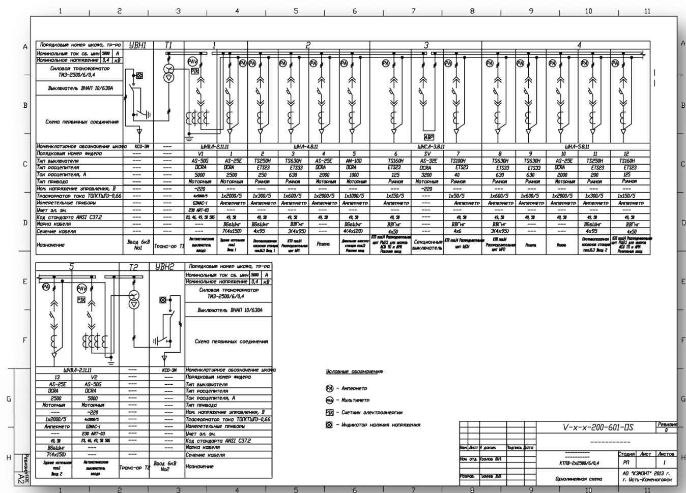
Рисунок 1 Пример заполнения однолинейной схемы
