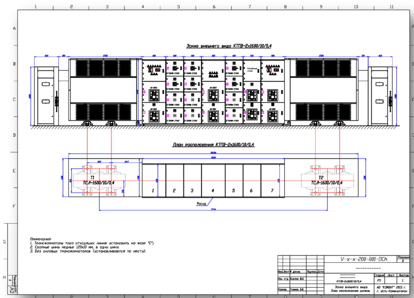
Рисунок 2 План расположения шкафов
